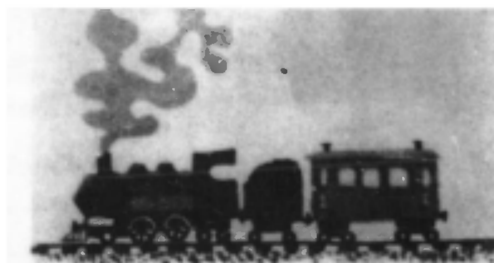
MAŞÎNA ŞEMANDEFÎRÊ
