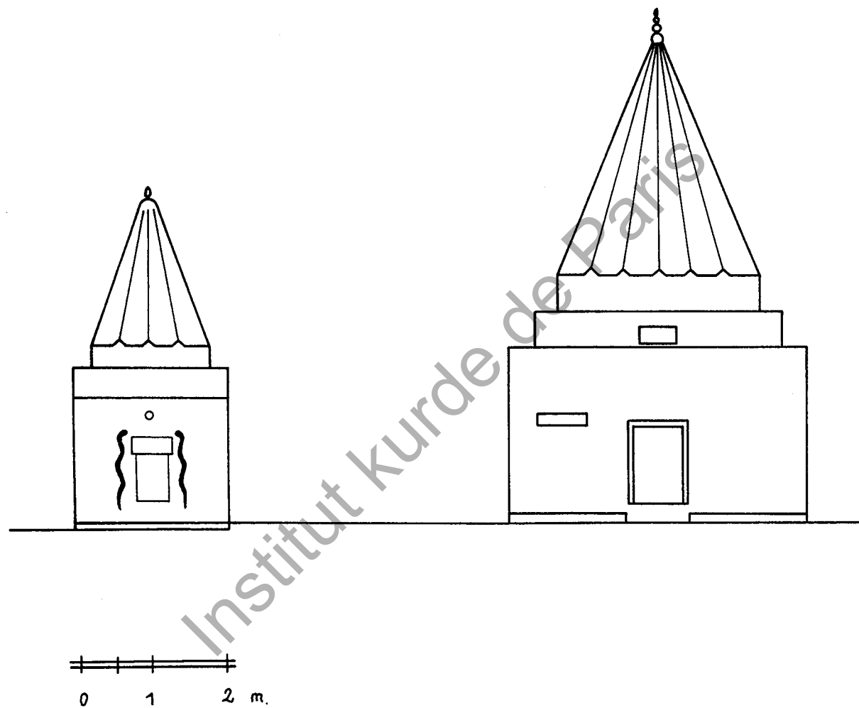
Planche 61 : Façades est des mausolées de Baba Çawuş et de Cheikh Mand Paşa, Kabartu.
