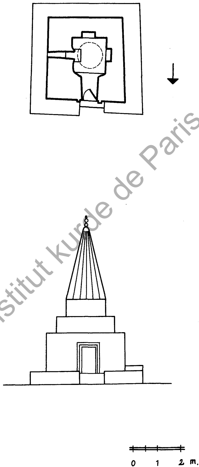
Planche 81 : Plan et façade nord du mausolée de Cheikh Barakât, Sindjar.
