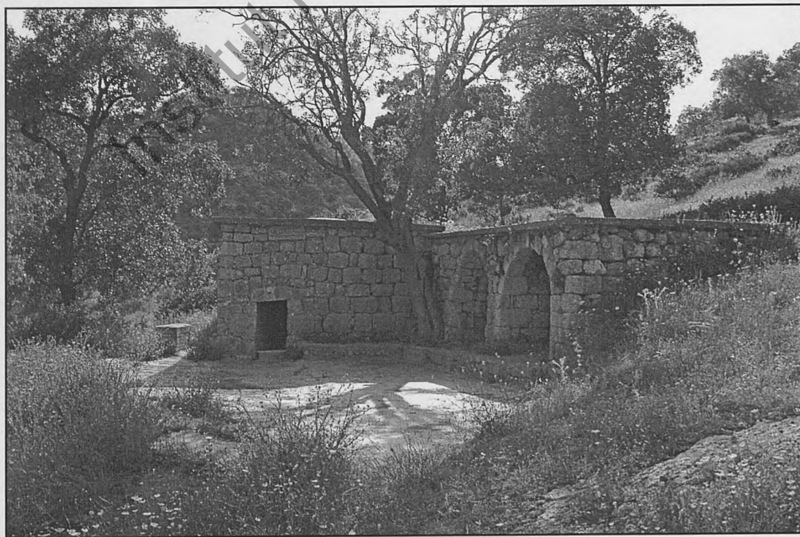
Figure 106 : Mausolée d'Alu Bekir, Laliş, vue vers l'ouest.
