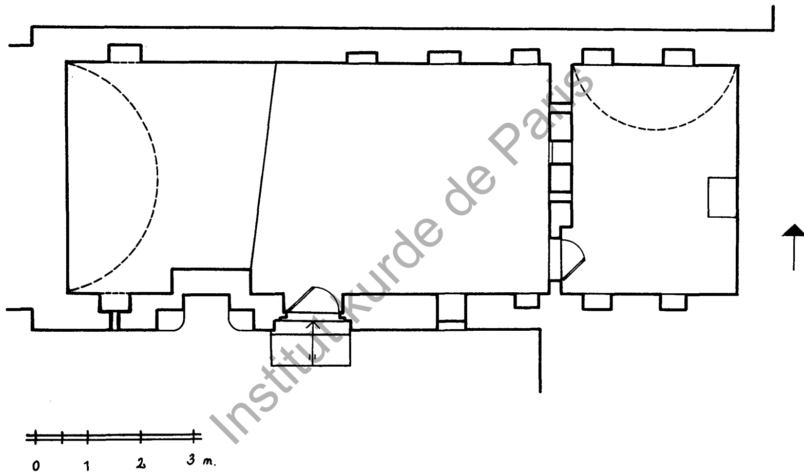
Planche 38. Plan du mausolée de Cheikh Şems, Bozan.
